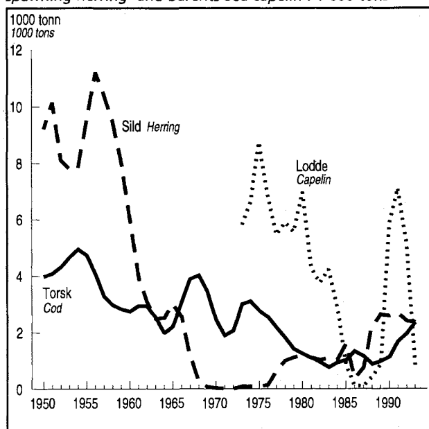
Figur 2.2. Bestandsutvikling for norsk-arktisk torsk 1 , norsk vårgytende sild 2 og lodde 3 i Barentshavet. 1 000 tonn
