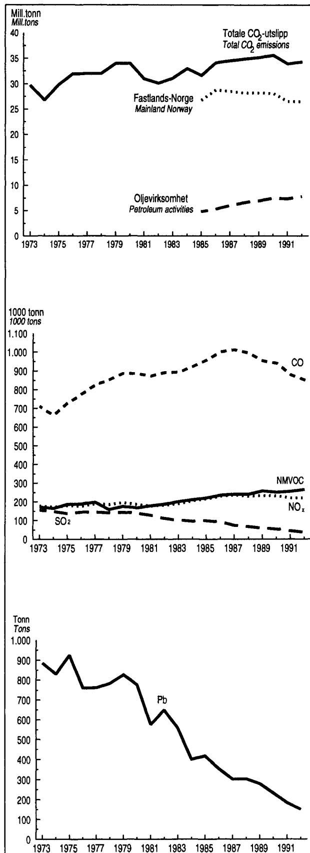
Figur 2.3. Utslipp til luft
