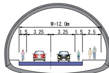
(トンネル部)
