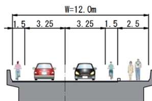
(橋梁部)
