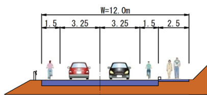
(土工部)
