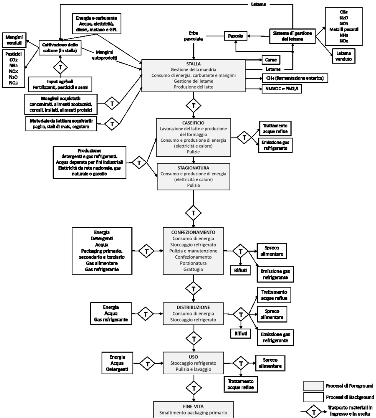
Figura 1 Diagramma di flusso delle fasi della filiera del Grana Padano DOP
