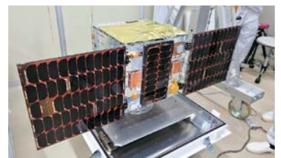
X線突発天体監視速報衛星「こよう」(金沢大学衛星1号機)
