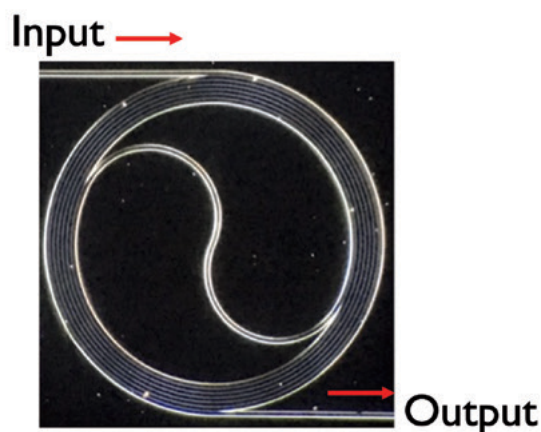
光AI回路チップ
