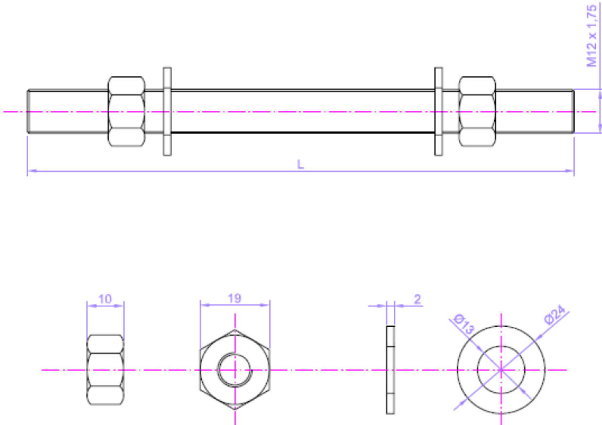
Figura 1 - Parafuso Prisioneiro M12 – Latão
