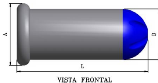
Figura 1 – Cartucho Metálico
