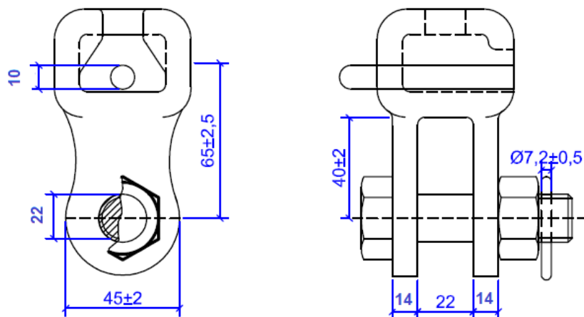
Figura 1 – Concha-Garfo 90°
