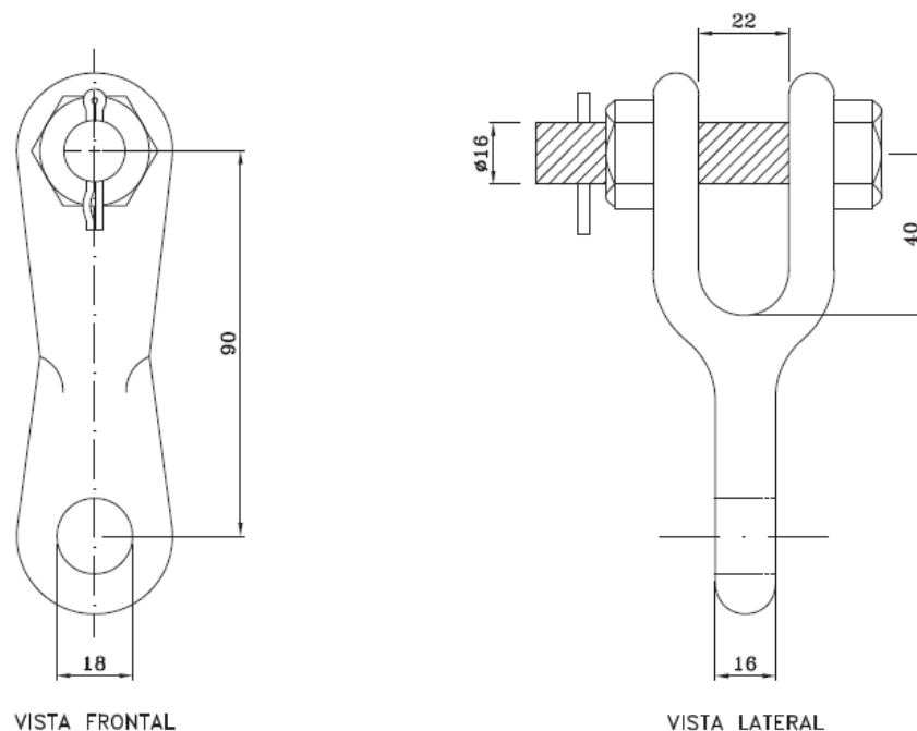
Figura 1 –Garfo-Olhal
