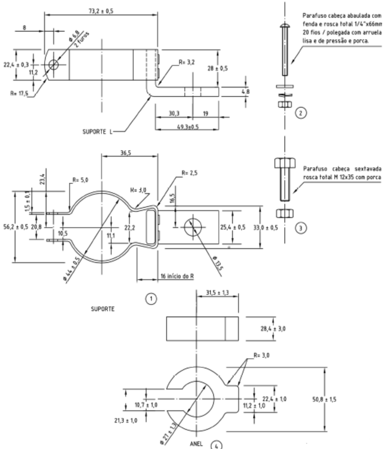
Figura 1 - Abraçadeira Para Cabo de Potência
