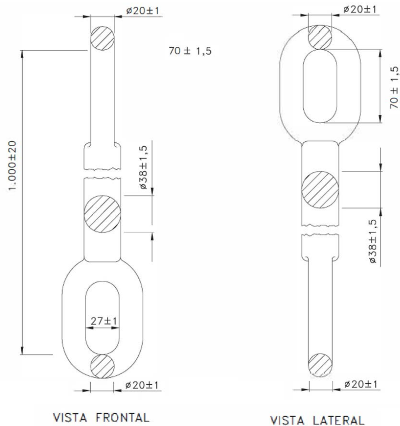
Figura 1 - Prolongador Elo-Elo 90°
