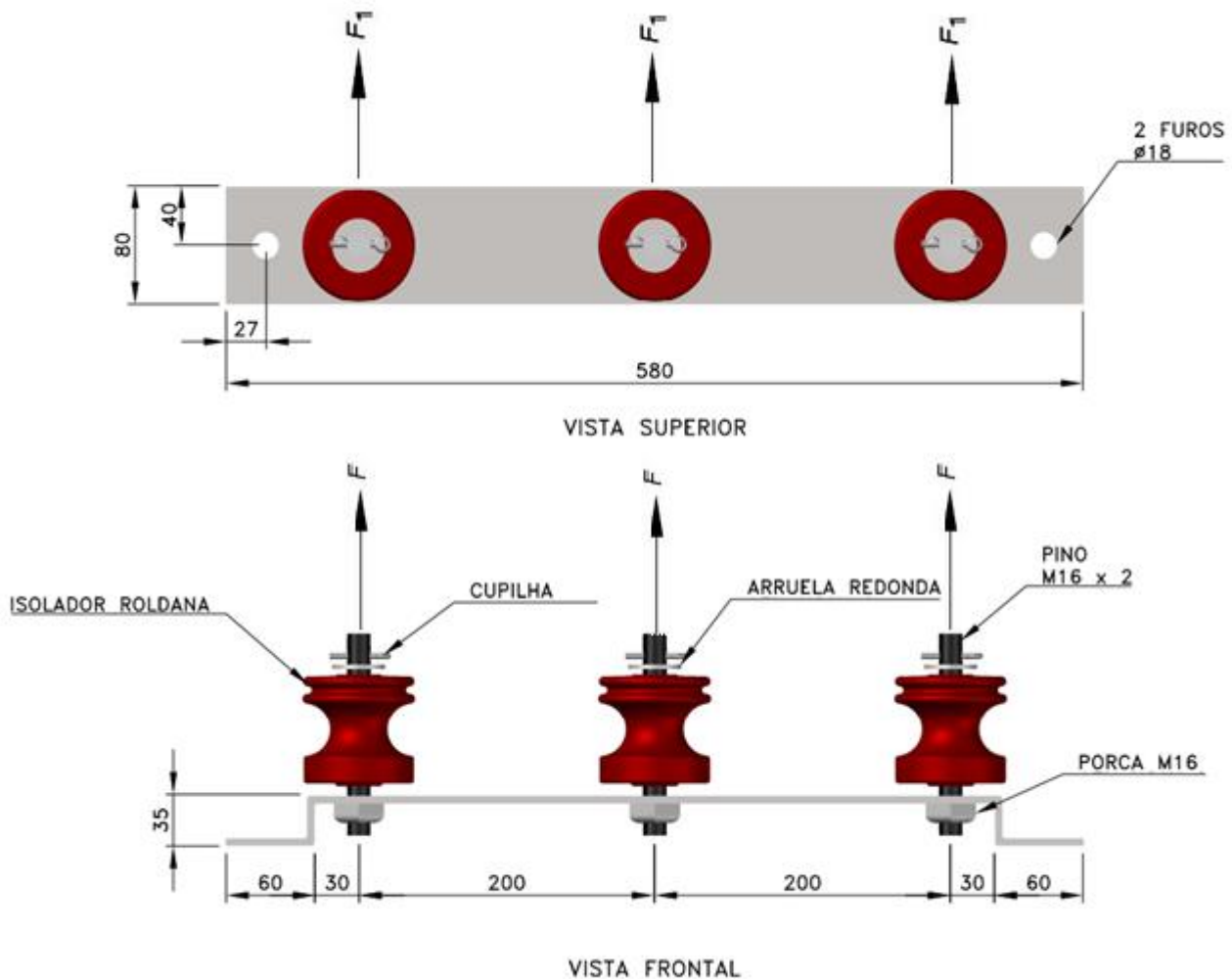
Figura 1 - Suporte para isolador roldana
