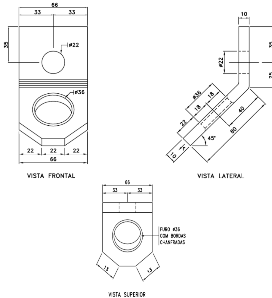
Figura 1 – Chapa Curva para Estai da Transmissão.
