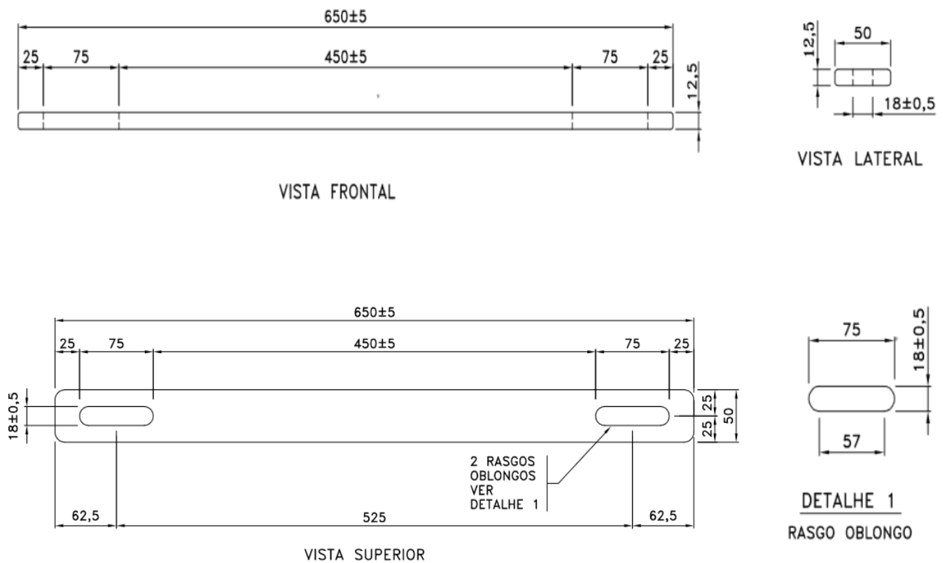
Figura 1 – Chapa de Fixação para Regulador de Tensão
