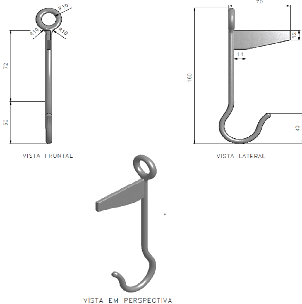
Figura 1 - Gancho para Olhal de Baixa Tensão – Monofásico e Trifásico
