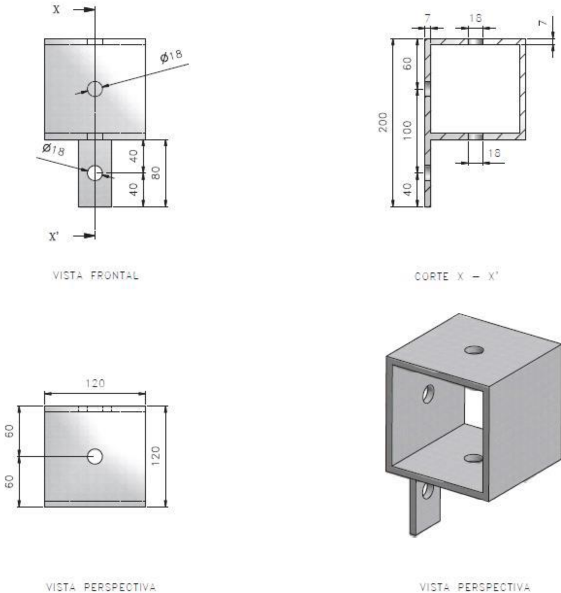
Figura 1 - Distanciador para Isolador Pilar
