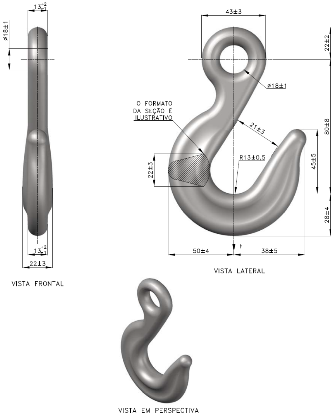
Figura 1 - Gancho Olhal
