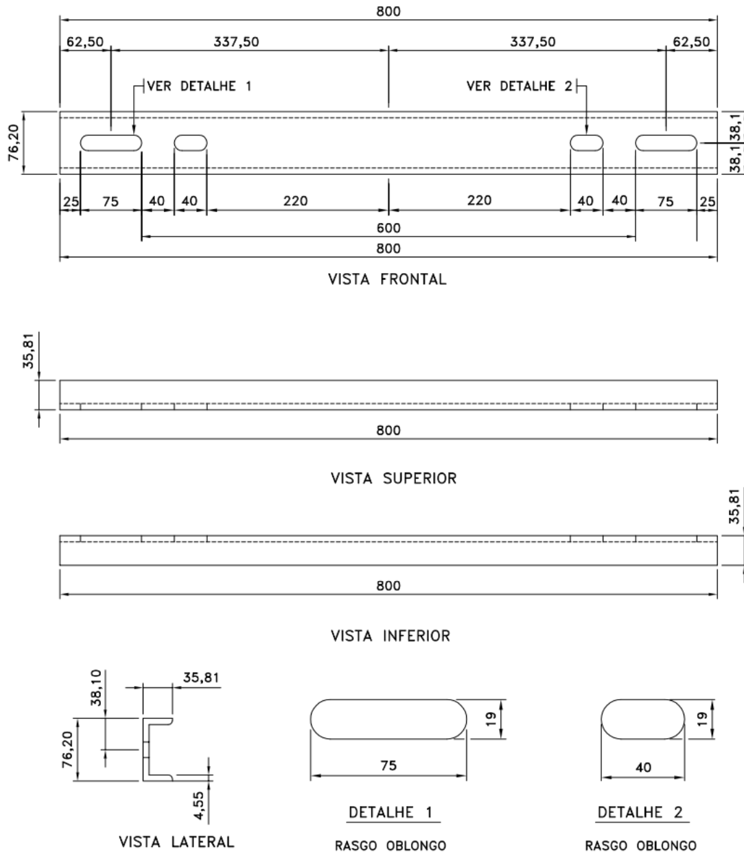
Figura 3 - Suporte Tipo 1, peça 3 – Fixação da base do regulador
