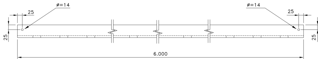
VISTA SUPERIOR
