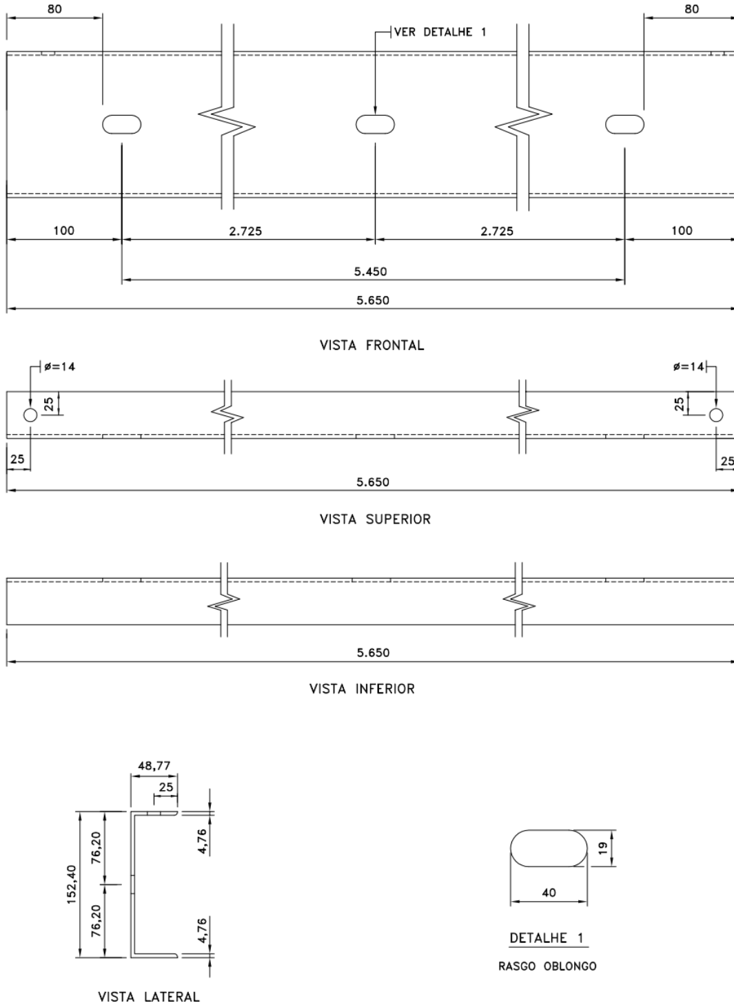
Figura 8 - Suporte tipo 3, peça 2 – Fixação das chaves
