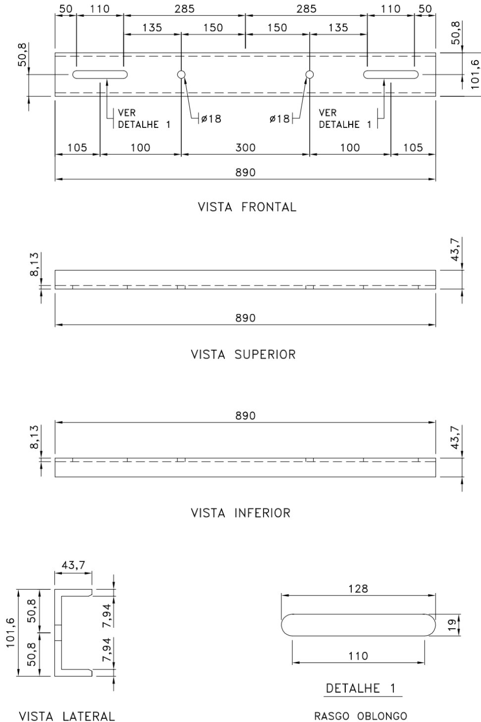
Figura 9 - Suporte Tipo 3, peça 3 – Fixação da base do regulador
