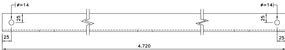
VISTA SUPERIOR
