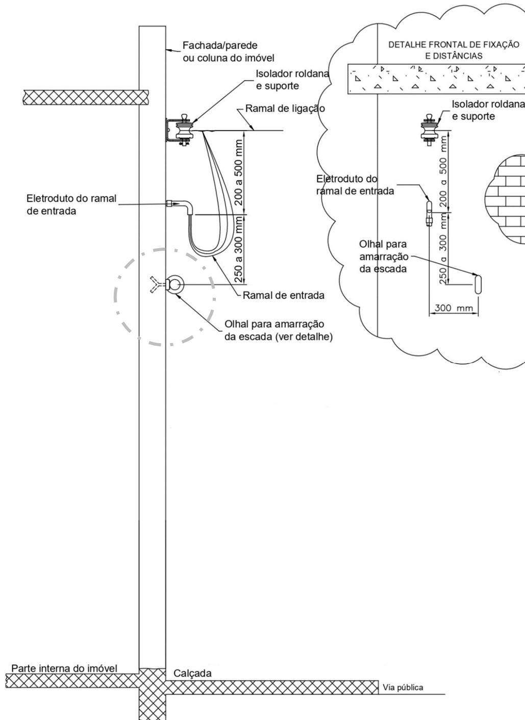
Figura 1 - Aplicação de olhal
