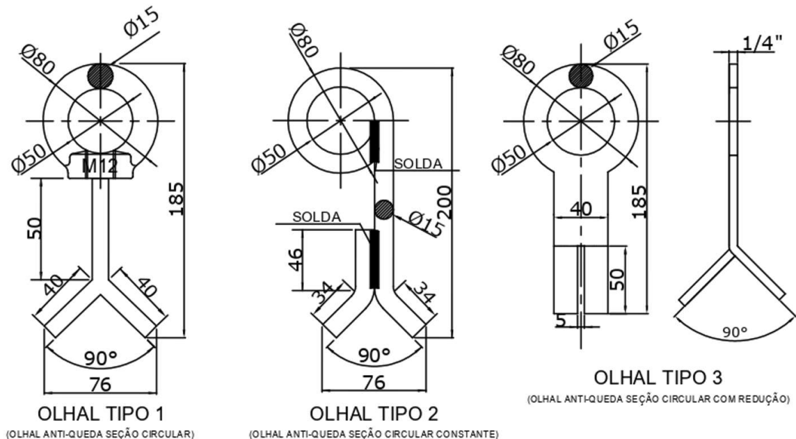
Figura 3 – Tipo de olhais - Aço inox
