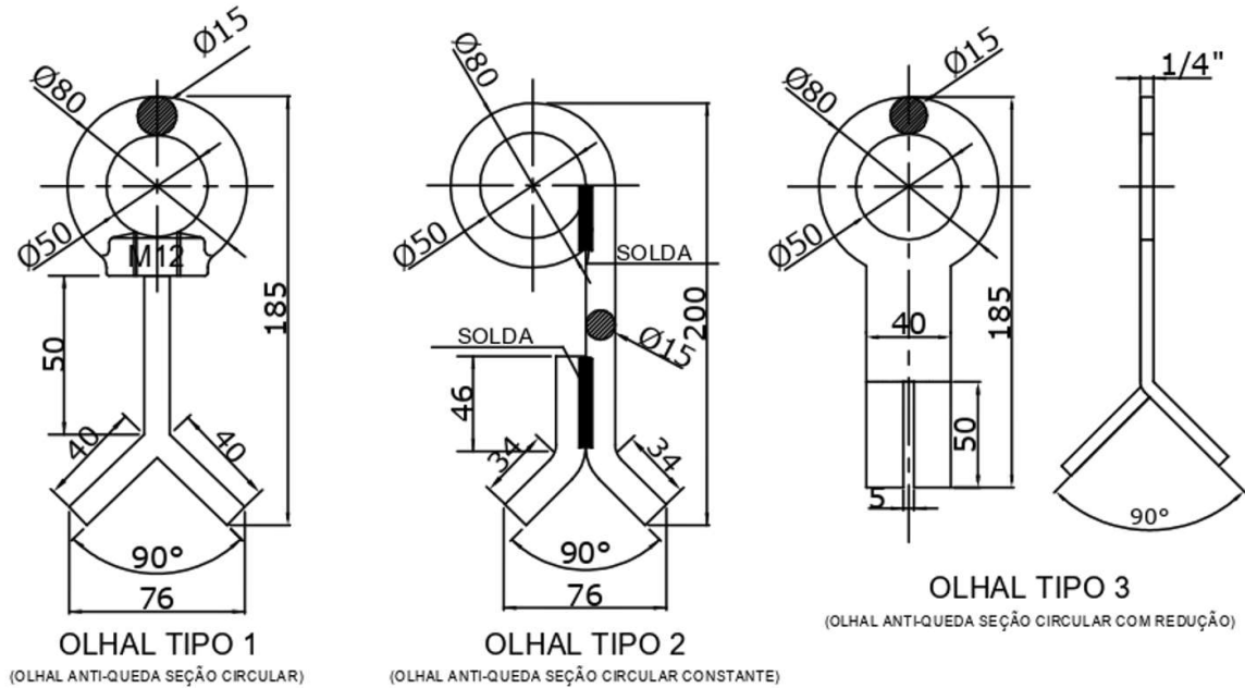
Figura 2 – Tipo de olhais- Aço galvanizado zincado;
