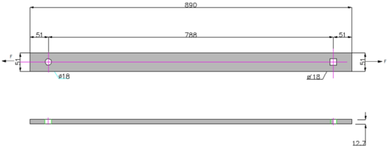
Figura 2 - Mão-Francesa Plana – Tipo 2
