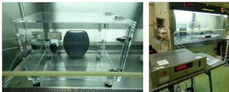
本研究における試験の様子 左:ボックス内でのオゾン曝露の様子、右:オゾン濃度モニターによる濃度制御
