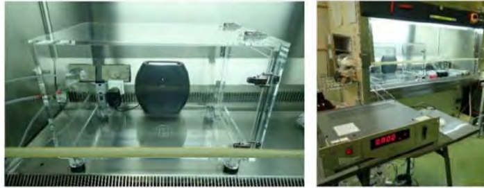
本研究における試験の様子 左:ボックス内でのオゾン曝露の様子、右:オゾン濃度モニターによる濃度制御
