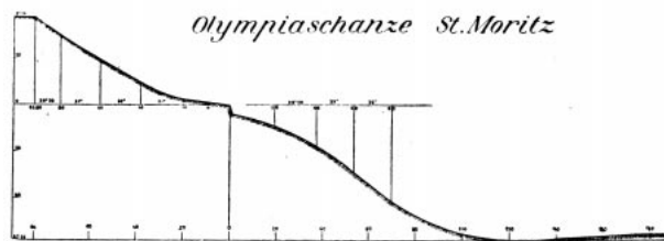
Profil du „tremplin de saut olympique“ de St-Moritz.
