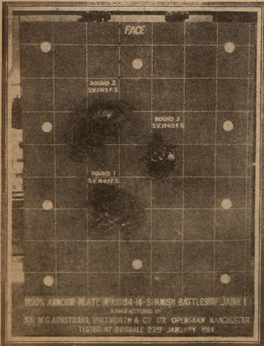
Часть поврежденной снарядами брони на борту англійскаго предноута. Для того, чтобы броня была пробита насквозь, снарядъ долженъ два-три раза попасть въ одно и то же мѣсто.
