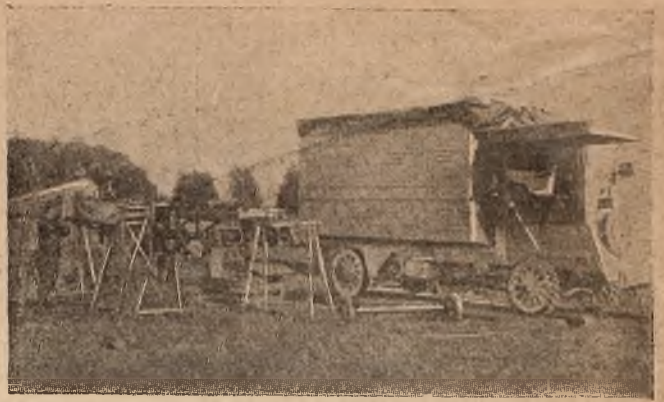
Специальные автомобили для перевозки въ сложенномъ видѣ аэроплановъ. Введены въ настоящее время въ англійской арміи.
