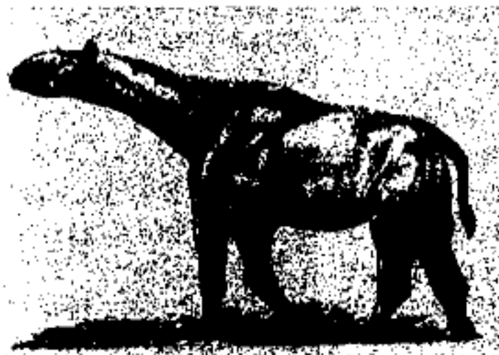
Индрикотерий (реконструкция)
