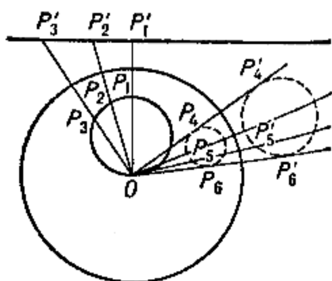
Инверсия
