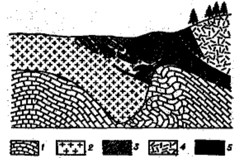
Геологический разрез. Разрез железорудного месторождения (Урал): 1 — известняки; 2 — сиениты; 3 — граниты; 4 — порфиры и туфы; 5 — магнитный железняк
