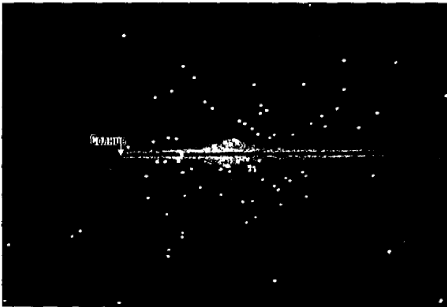
Галактика. Схематическое изображение (вид с ребра)
