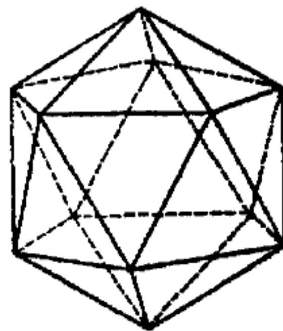
Икосаэдр
