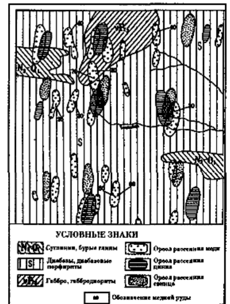
Геохимическая карта (фрагмент)
