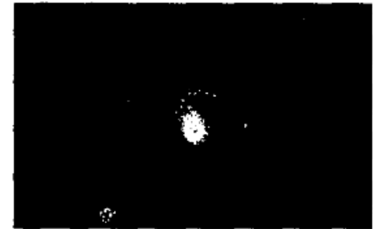
Спиральные Галактики
