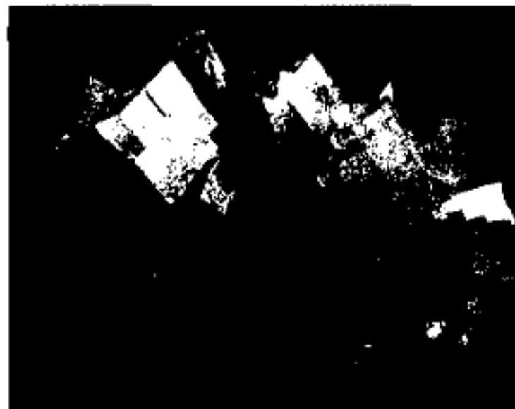
Галит
