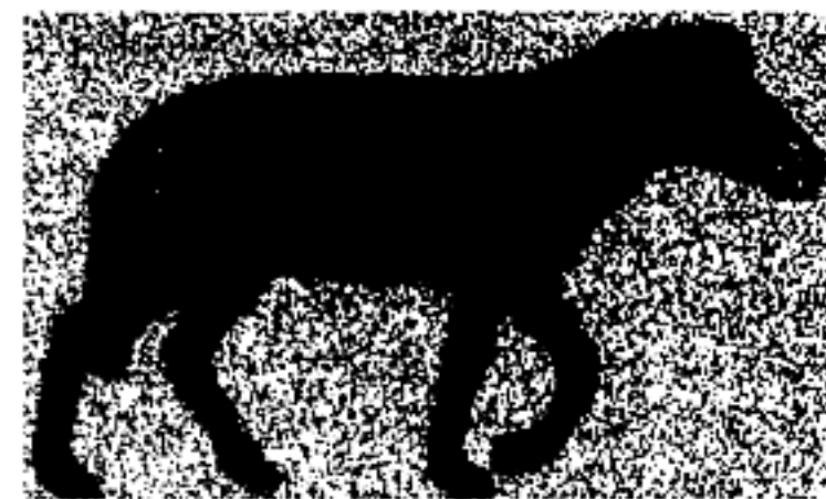
Гиппарион
