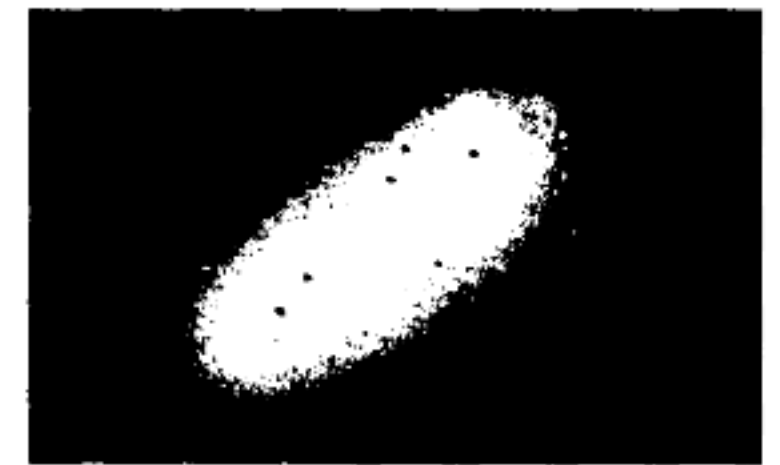
Эллиптические Галактики
