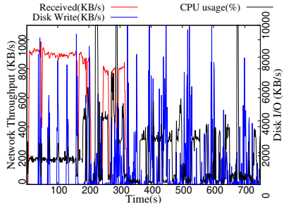
(d) BigLayers image with a 1 Mbps network cap.
