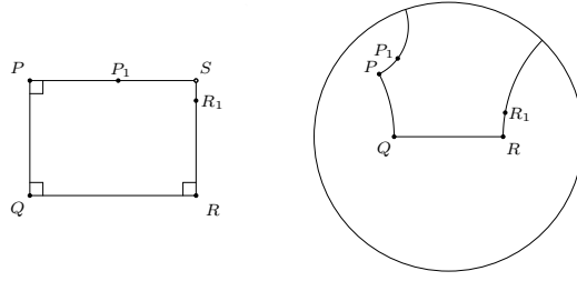
Fig. 16: Bachmann's Lotschnittaxiom (Postulate 4).
