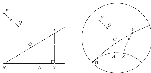
Fig. 17: Aristotle's axiom (Axiom 3).
