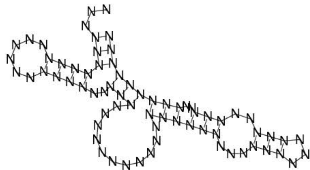
Input Motif
