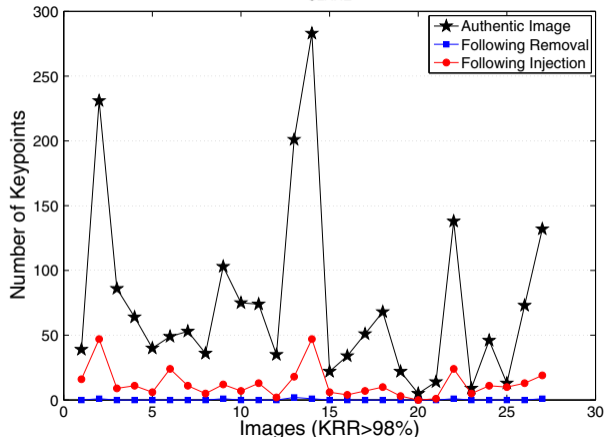
CLAHE
