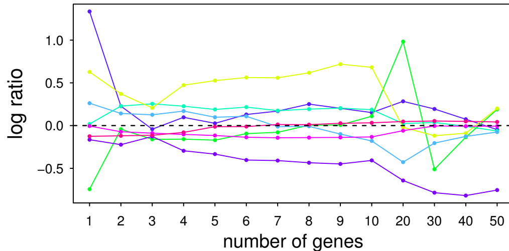
(KNN)
