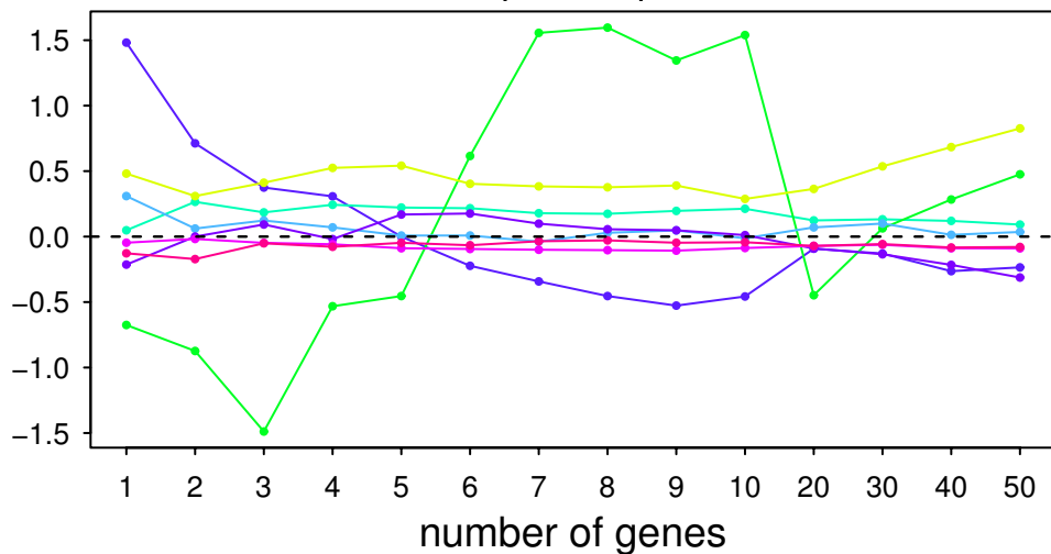
(SVM)
