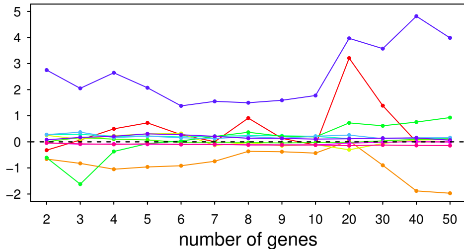
(RF)
