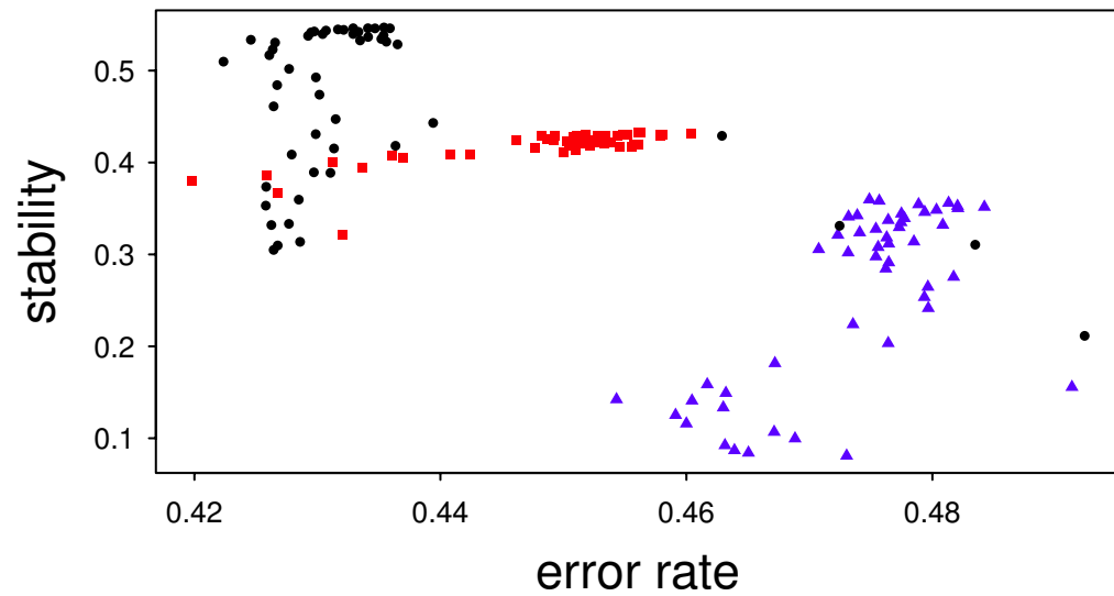
KNN
