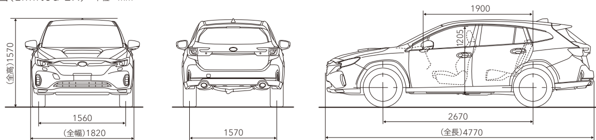
3面図(Limited EX) 単位: mm
