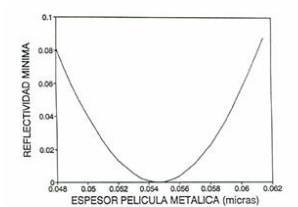
Fig. 3. Determinación del espesor óptico h_{opt} de la película metálica en la configuración de Kretschmann. Graficamos el mínimo de la reflectividad como función del espesor h_2 de la película metálica (en micras). El valor mínimo de la reflectividad se encuentra en h_{opt}=0.054\mu m .
