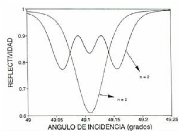
Fig. 7. Influencia de la forma del haz incidente en la excitación del plasmón de superficie de largo alcance de la configuración de Sarid. El haz incidente es un haz Hermite-Gauss, con n=2 y ancho L=200\mu m . Se presenta también el resultado de un haz incidente gaussiano ( n=0 ) del mismo ancho.
