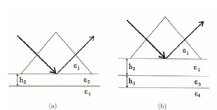
Fig. 2. En la figura (a) mostramos la configuración de Kretschmann, y en la figura (b) la propuesta por Sarid para la excitación de plasmones de largo alcance.
