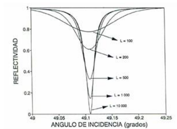
Fig. 6. Influencia del ancho L de un haz gaussiano incidente en el acoplamiento con el plasmón de superficie de largo alcance en la configuración de Sarid. Se consideran los siguientes anchos: L=10000\mu\text{m} (onda plana), L=1000\mu\text{m} , L=500\mu\text{m} , L=200\mu\text{m} y L=100\mu\text{m} . Los espesores de las películas dieléctrica y metálica son h_2=1.28\mu\text{m} y h_3=0.0170\mu\text{m} , respectivamente. Compare el ancho angular de las resonancias con los de la configuración de Kretschmann en la Fig. 4.
