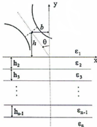
Fig. 1. Nuestro sistema consta de n películas homogéneas paralelas al plano OXZ. Cada película se caracteriza por su espesor h_j y su permitividad compleja \epsilon_j , con j=1, \dots, n . El espesor del sustrato y el superestrato es infinito. Un haz incide del medio 1 con un ángulo de inclinación \theta_0 .
