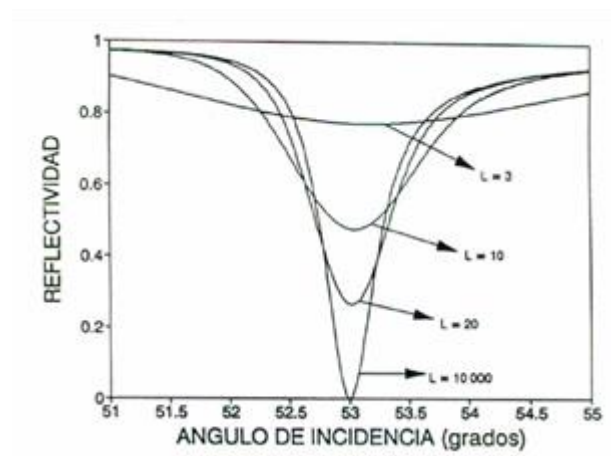
Fig. 4. Influencia del ancho L de un haz gaussiano incidente en el acoplamiento con el plasmón de superficie obtenido con la configuración de Kretschmann. Se consideran los siguientes anchos: L = 10000\mu\text{m} (onda plana), L = 20\mu\text{m} , L = 10\mu\text{m} y L = 3\mu\text{m} . El espesor de la película metálica es h_{opt} = 0.0546\mu\text{m} .
