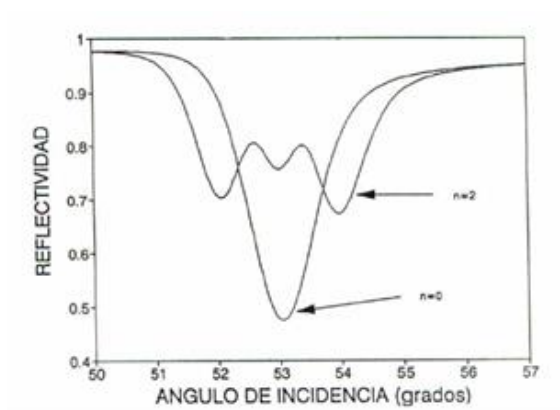
Fig. 5. Influencia de la forma del haz incidente en la excitación del plasmón de superficie de la configuración de Krestchmann. El haz incidente es un haz Hermite-Gauss, con n=2 y ancho L=10\mu\text{m} . Se presenta también el resultado de un haz incidente gaussiano ( n=0 ) del mismo ancho.
