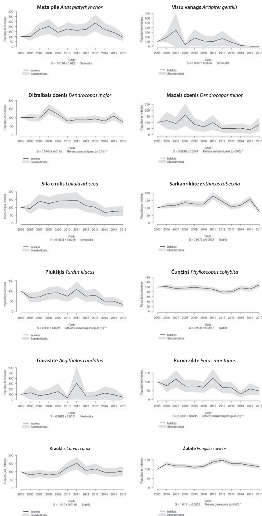
3. ATTĒLS. Dažu sugu populāciju indeksi 2005.–2016. gadu periodā. FIGURE 3. Population indices of selected species 2005–2016.
