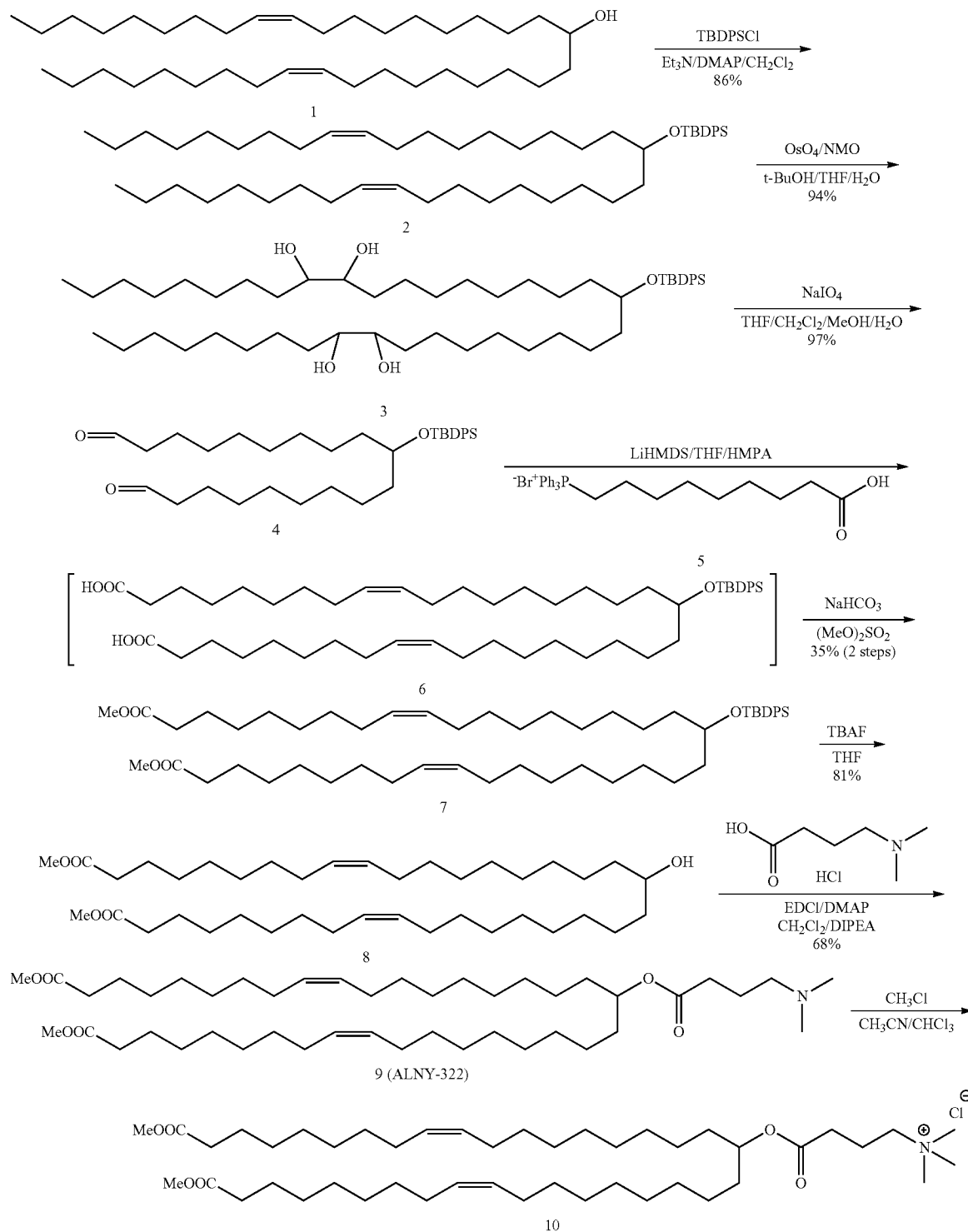
Scheme 1. ALNY-322/quaternary salts
