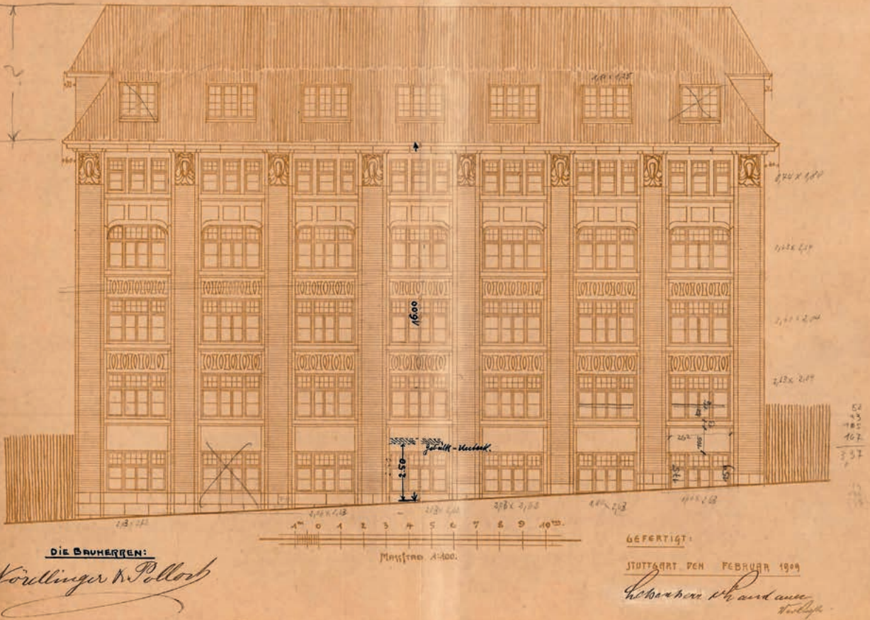
Abb. 14 Lehnherr & Landauer: Fassadenentwurf Reuchlinstr. 4b vom Februar 1909
