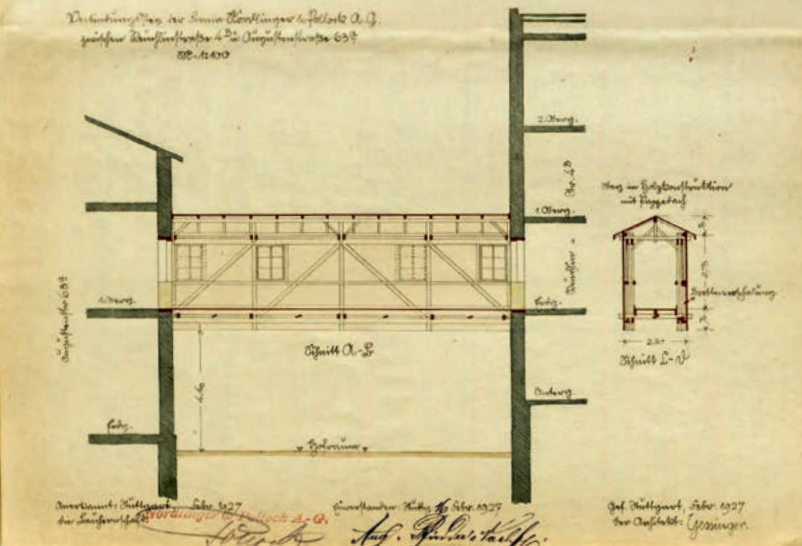
Abb. 27 Paul Gessinger: Aufriss des hölzernen Verbindungsganges zwischen dem Erweiterungsbau und dem Nachbargebäude vom Februar 1927
