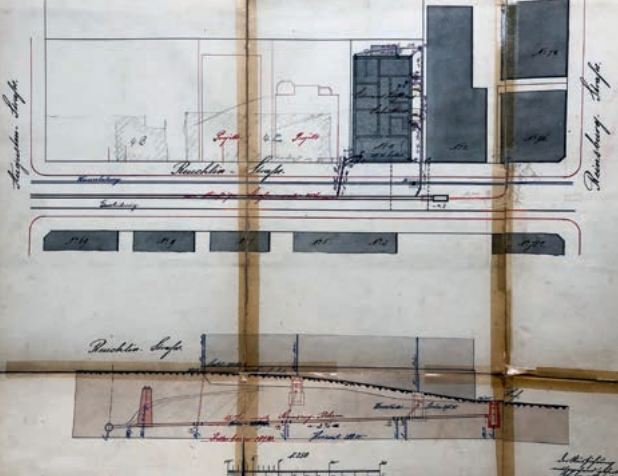
Abb. 2 Kanalisationsplan der Reuchlinstraße vom August 1882
