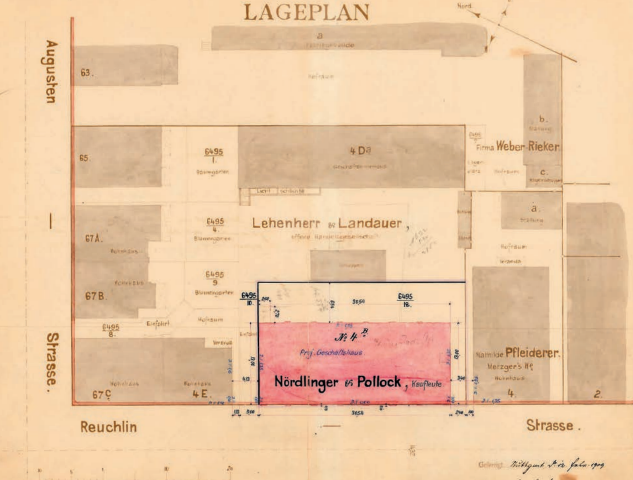
Abb. 4 Lehenherr & Landauer: Lageplan des projektierten Geschäftshauses Nördlinger & Pollock vom 12. Februar 1909
