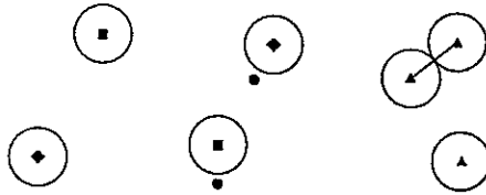
Figura 5.1: A figura representa uma instância (G, c, \{R_1, R_2, R_3\}) do MINFS. O grafo G é completo e tem 9 vértices. As arestas estão implícitas; o custo c_e de cada aresta e é a distância euclidiana entre os extremos de e . Os elementos de R_1, R_2 e R_3 estão representados por triângulos, losangos e quadrados.
