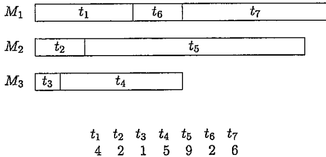
Figura 2.1: Exemplo de escalonamento com 7 tarefas em 3 máquinas. A duração da tarefa i é t_i . O critério de Graham produz o escalonamento \{\{1, 6, 7\}, \{2, 5\}, \{3, 4\}\} , representado na figura. Esse escalonamento tem custo t_1 + t_6 + t_7 = 12 . Um outro escalonamento é \{\{1, 7\}, \{2, 4, 6\}, \{3, 5\}\} , que tem custo t_3 + t_5 = 10 .
