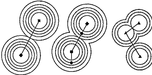
Figura 5.5: Início da sexta iteração.
