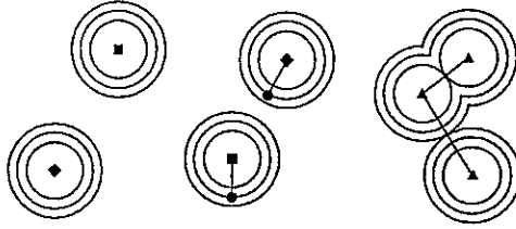
Figura 5.4: Situação no início da quinta iteração.
