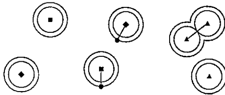
Figura 5.3: Situação no início da quarta iteração. As arestas da floresta F são indicadas por linhas sólidas. (Continua na próxima figura.)
