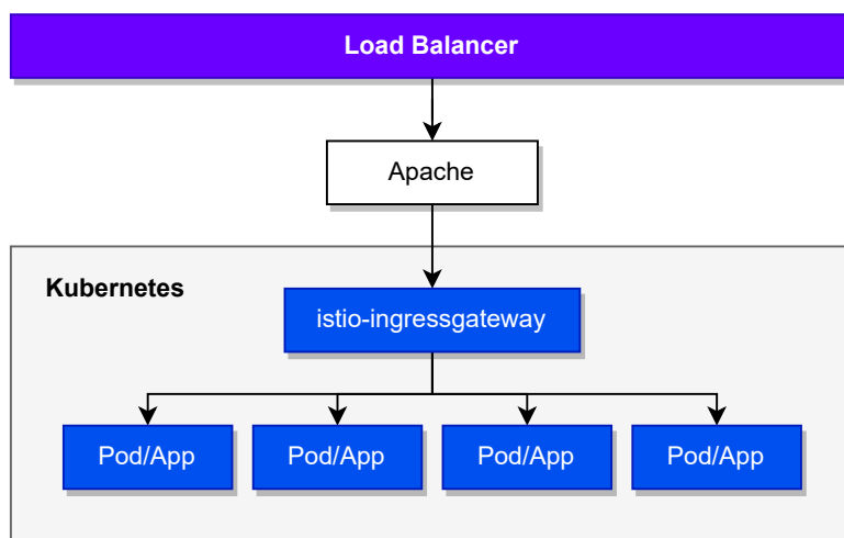
図 4: 移行時のネットワーク構成
