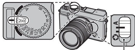
Diafragmastandenschakelaar
