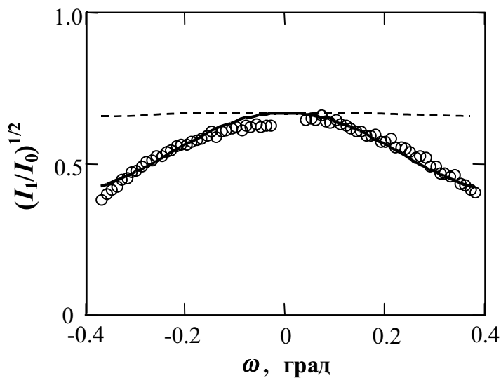
Рис.2. Экспериментальные данные (кружки) и теоретической расчеты в Борновском приближении метода искаженных волн для случая полной кросс-корреляции шероховатостей (пунктир) и сглаживания шероховатостей (сплошная линия).
