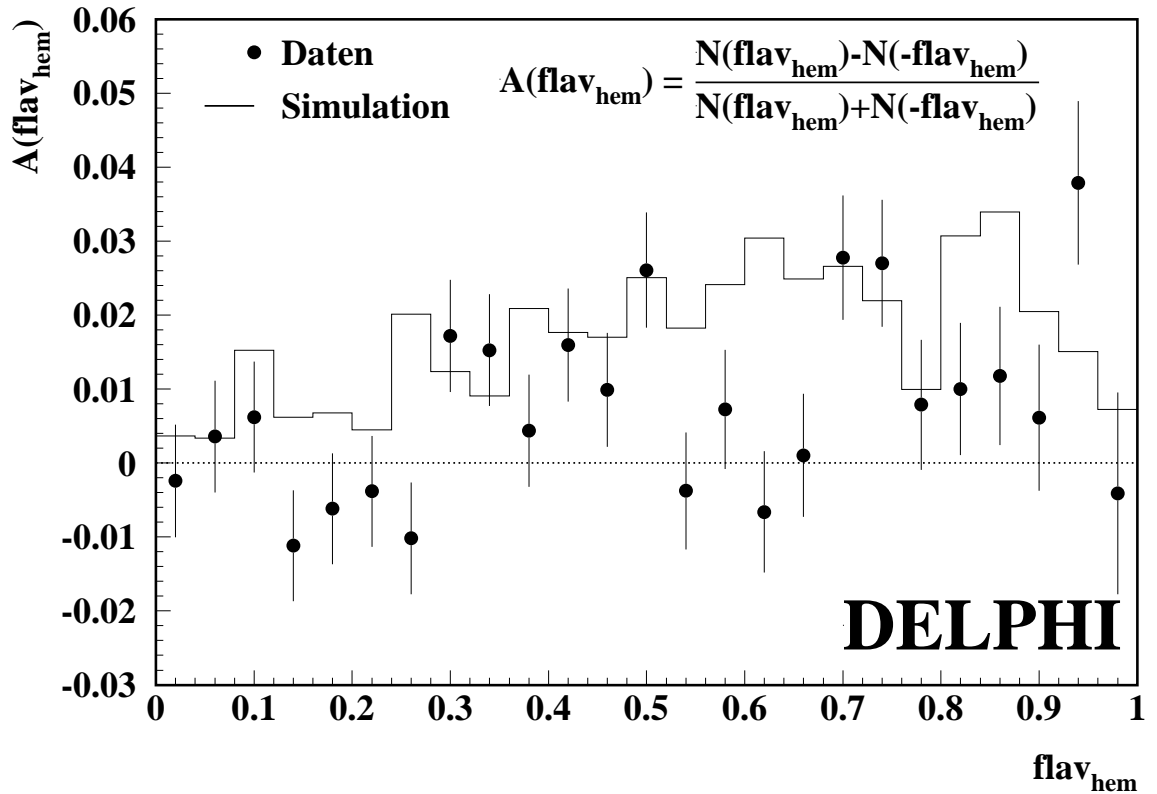
Abbildung 5.6: Die Asymmetrie der flav_{\text{hem}} -Verteilung wird für Daten und Simulation für 1994 verglichen. Die flav_{\text{hem}} -Verteilung ist nicht spiegelsymmetrisch bezüglich der Spiegelung um die y -Achse der Verteilung (Abbildung 4.19), sondern zeigt eine kleine Asymmetrie. Angewendeter Selektionsschnitt: b_{\text{tag},1994-1995} > 0.1
