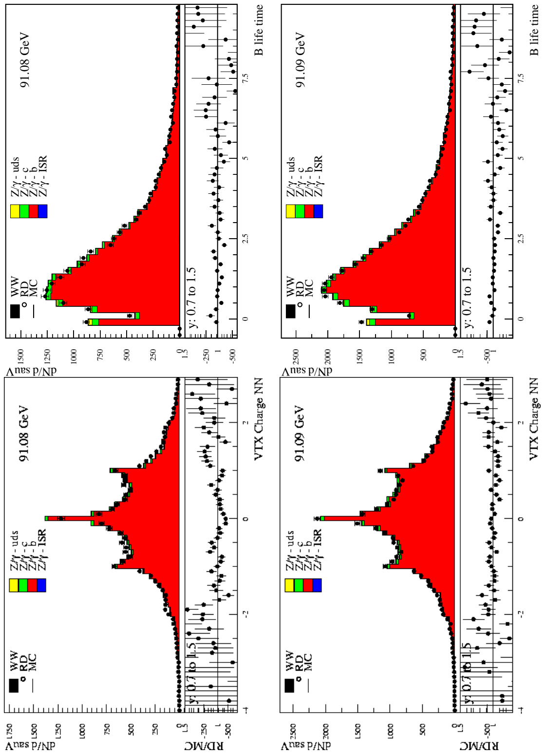
Abbildung B.8: Vergleich zwischen der alten (links) und der neuen (rechts) BSAURUS-Version für die Vertexladung (unten) und die B -Lebensdauer (oben) [84]. Der verwendete Signalebereich wird durch den Selektionsschnitt b_{\text{tag}} > 0.5 definiert.
