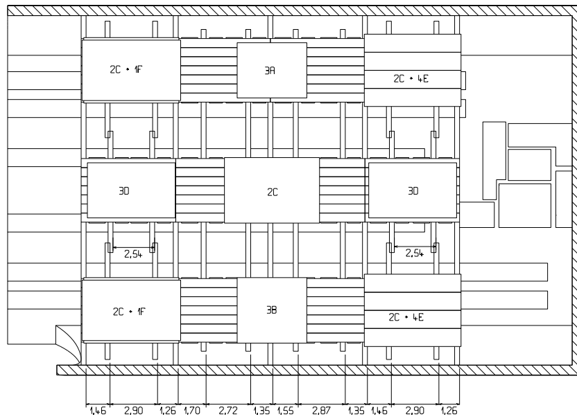
Vue en plan du montage des detecteurs
