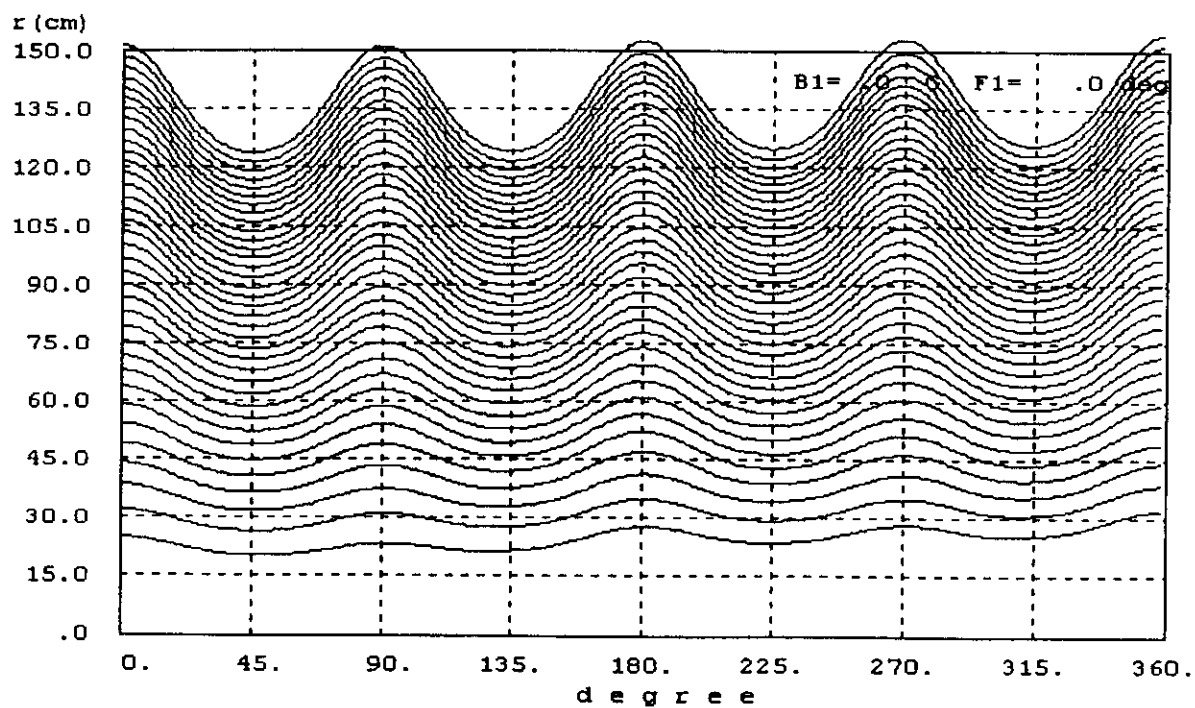
Рис. 12. Радиальные траектории центральной частицы фазового объема пучка в течение 36 оборотов
