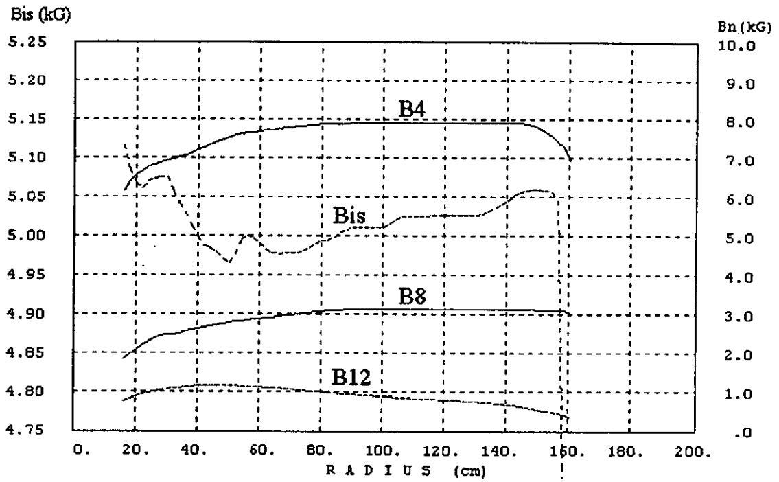
Рис. 1. Характеристики магнитного поля
