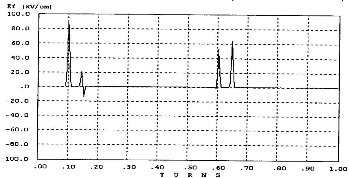
Рис. 8. Напряженность ускоряющего поля на первом обороте для частицы с оптимальными начальными условиями
