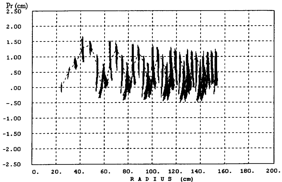
Рис. 13. Характеристики ускорения центральной частицы фазового объема пучка
