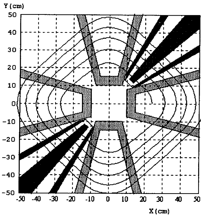
Рис. 6. Пять оборотов частицы с оптимальными начальными условиями
