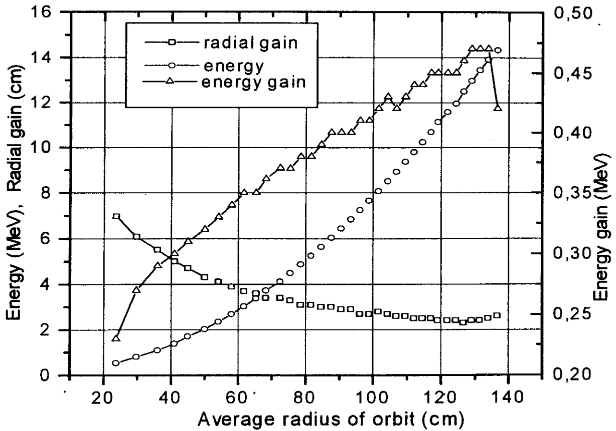
Рис. 13. Характеристики ускорения центральной частицы фазового объема пучка
