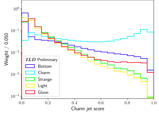
(b) c -jet score
