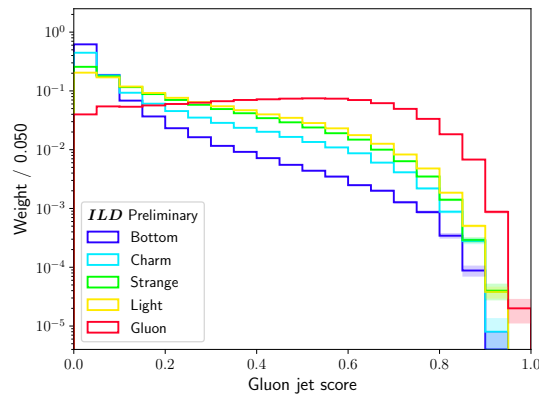
(e) g -jet score
