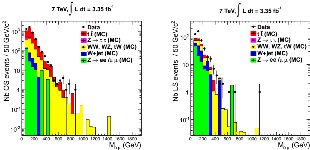
FIG. 8.6 – Distributions du spectre de masse invariante des paires e\mu (à gauche) de charges opposées et (à droite) de même charge, pour les données et les simulations.
