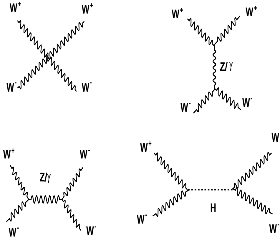
FIG. 1.5 – Diagrammes de Feynman pour le processus W^+W^- \rightarrow W^+W^-
