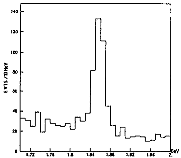
(d) D^+ \rightarrow K^- \pi^+ \pi^+ ( N_\sigma > 4 ).
