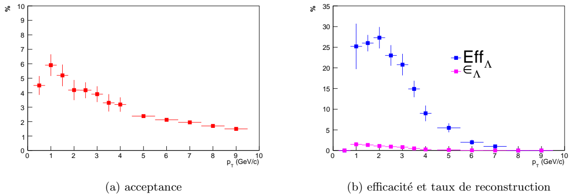
FIG. 5.3 – Acceptance, efficacité et taux de reconstruction des \Lambda en fonction du p_T dans une zone fiduciaire restreinte 0.9 < r_{\perp} < 2.9 cm.
