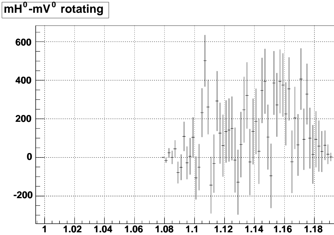
FIG. A.4 – Spectre de m_{\Lambda p \pi^-} - m_{\Lambda} pour les coupures du tableau A.2.
