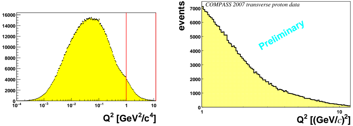
FIG. 4.6 – Distribution de la variable Q^2 pour 2004 (à gauche) et 2007 (à droite). Toutes les coupures sont appliquées sauf la coupure sur Q^2 pour la figure de 2004, la coupure en Q^2 est appliquée pour 2007.
