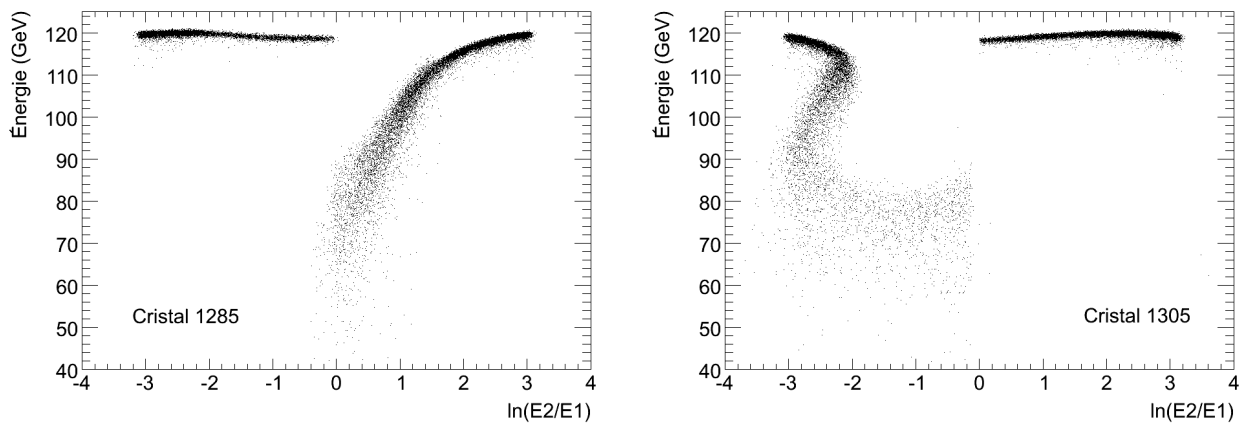
FIG. 6.77: Énergie mesurée dans une somme de 9 cristaux en fonction de \ln(\frac{E_2}{E_1}) selon la direction \eta , pour le cristal 1285 (à gauche) et pour le cristal 1305 (à droite), obtenue avec des données simulées où le faisceau de 120 GeV est centré au milieu et sur les bords gauches et droits du cristal.
