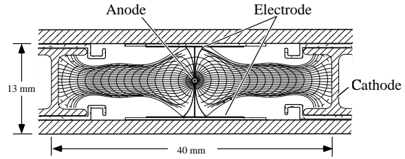
FIG. 4.14: Coupe transverse d'un tube à dérive (DT)
