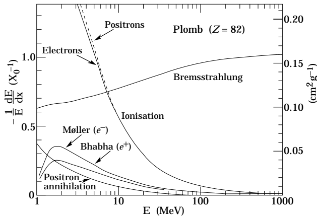
FIG. 5.3: Fraction d'énergie perdue par un électron, ou un positron, par longueur de radiation X_0 , dans le cas du plomb. Le bremsstrahlung domine tous les autres processus à partir de \approx 10 \text{ MeV} [30]. À 100 MeV un électron (ou positron) perd, par rayonnement de freinage, plus de 90% de son énergie par unité de X_0 .
