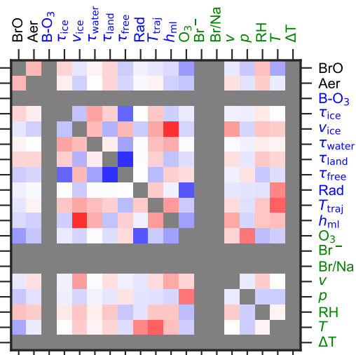
(d) NDJ
