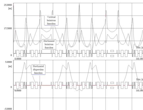
Figure 2: Twiss parameter of CSRm
